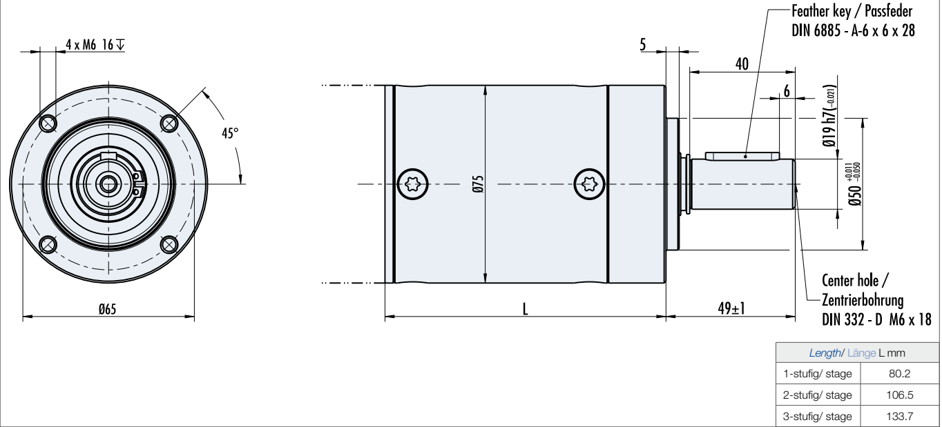
Dimensions in mm/ Maßzeichnung in mm
