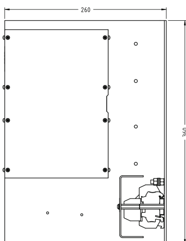
B1591-30-FRONT
