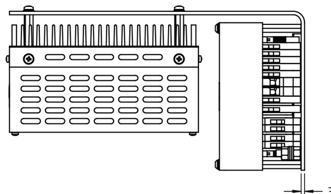
B1591-30-TOP
